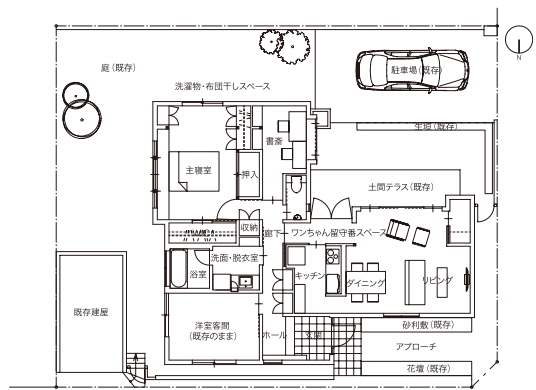
1階平面 縮尺1/300
