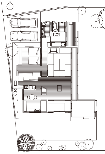
1階平面 縮尺1/300
